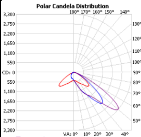
配光曲線
